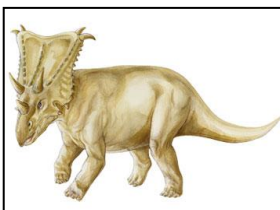
Chasmosaurus
